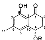
(4S)-shinanolone ( 5 ) R=H ( 5s ) R=(S)\text{-MTPA} ( 5r ) R=(R)\text{-MTPA}
