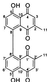
maritinone ( 2 )
